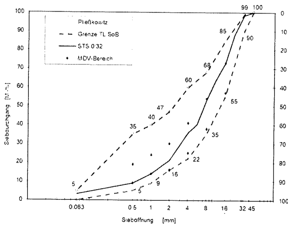
Baustoffgemisch STS 0/32 und Sieblinienbereich für STS 0/32 gemäß TL SoB-StB
